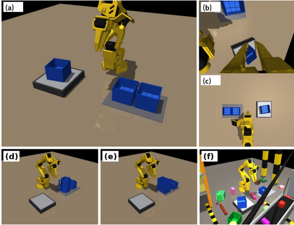
그림 2. 시뮬레이션 셀 (a) 전체 (b) 손목 카메라 (c) 상단 카메라 (d) 컵 (e) 직사각형 상자 (f) 공장형 환경
