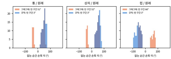
그림 3. 잡는 순간의 손목 회전각 (1 층 시연): 사람식(주황)은 두 무리로 갈리고 R2(파랑)는 연속으로 퍼진다
