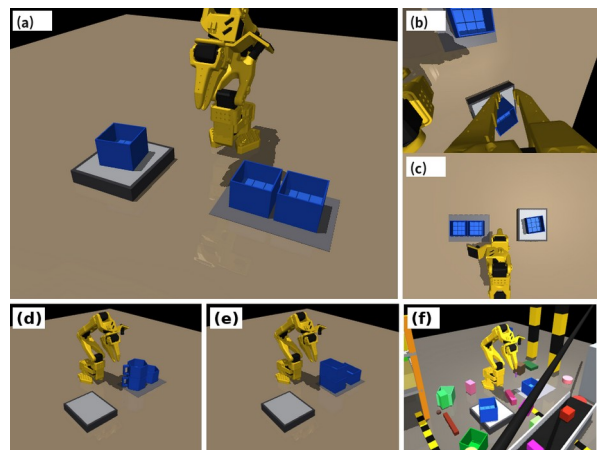
그림 2. 시뮬레이션 셀 (a) 전체 (b) 손목 카메라 (c) 상단 카메라 (d) 컵 (e) 직사각형 상자 (f) 공장형 환경
