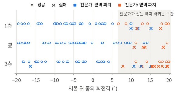
그림 3. 저울 위 통의 회전각과 단계별 결과 (여유 9mm, 로봇 쪽 벽, 시연 100)
