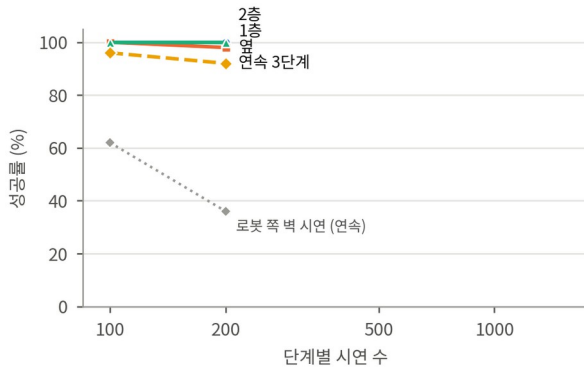
그림 4. 시연 수에 따른 적재 성공률 (④ 시연)
