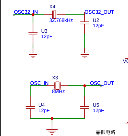
晶振电路
