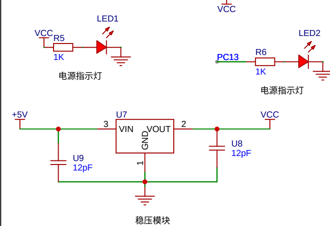
稳压模块
