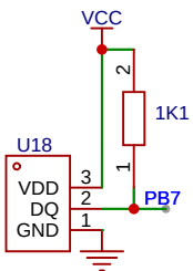
DS18B20
