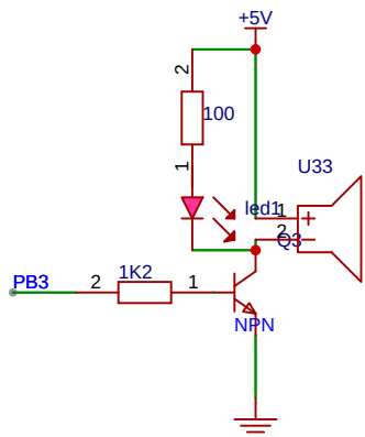
有源蜂鸣器
