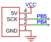
HX711压力传感器
