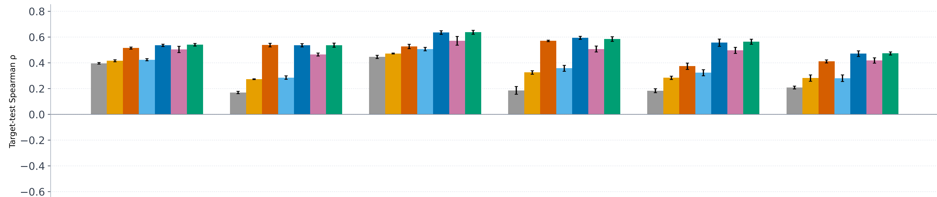
MLP
