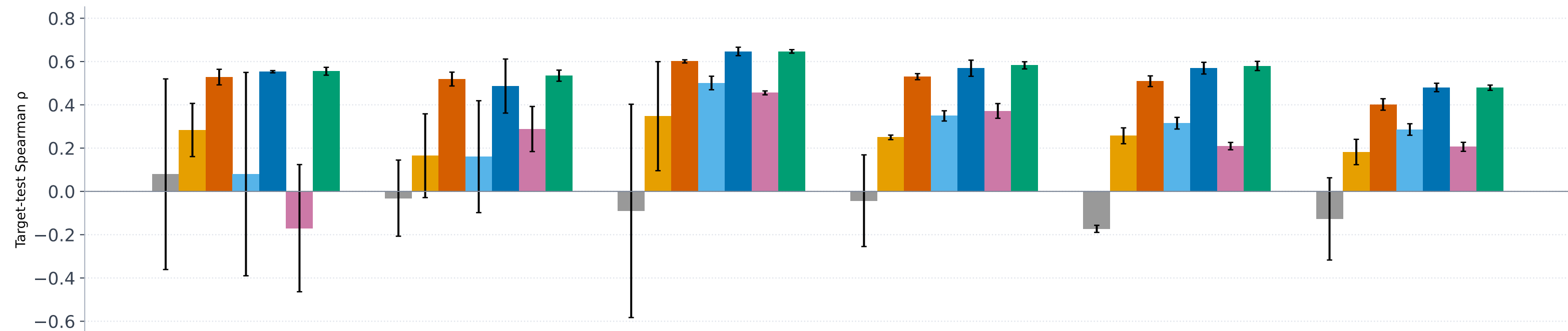
Linear
