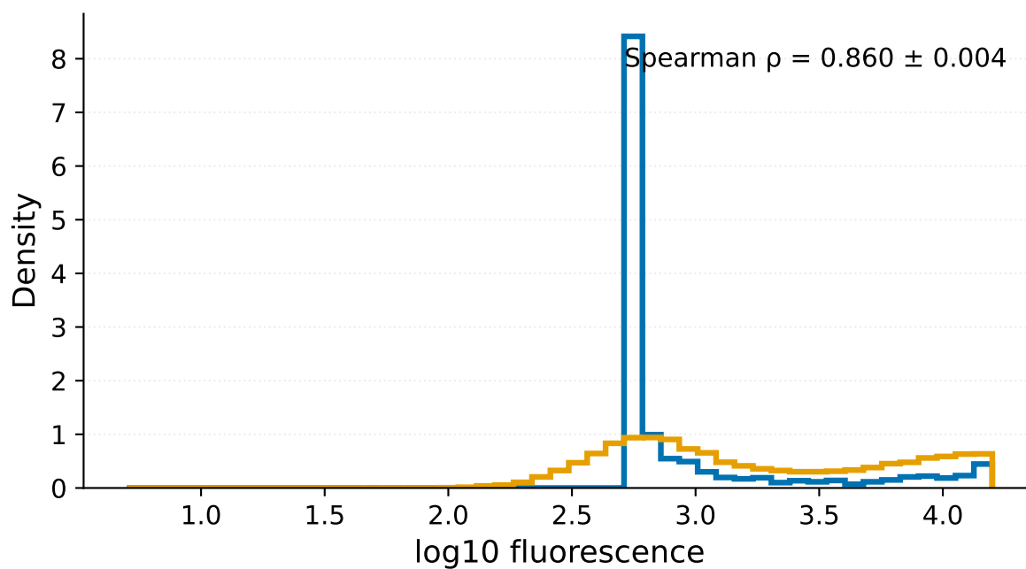
MLP
