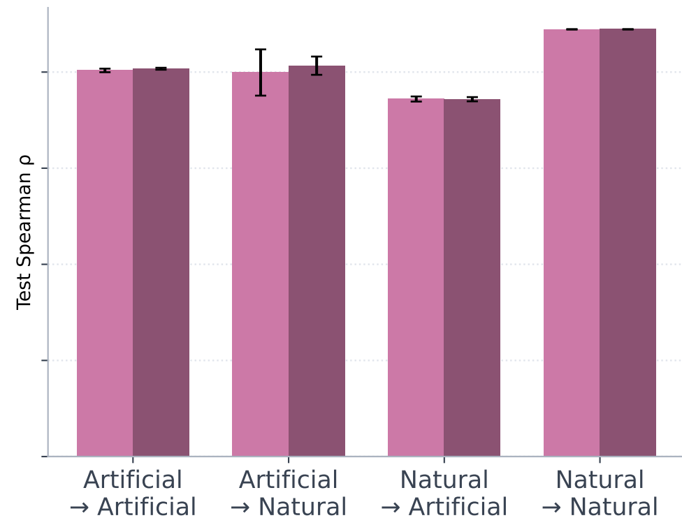
MLP
