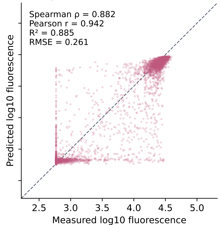
CNN Jannis
