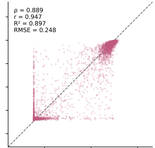
CNN Jannis
