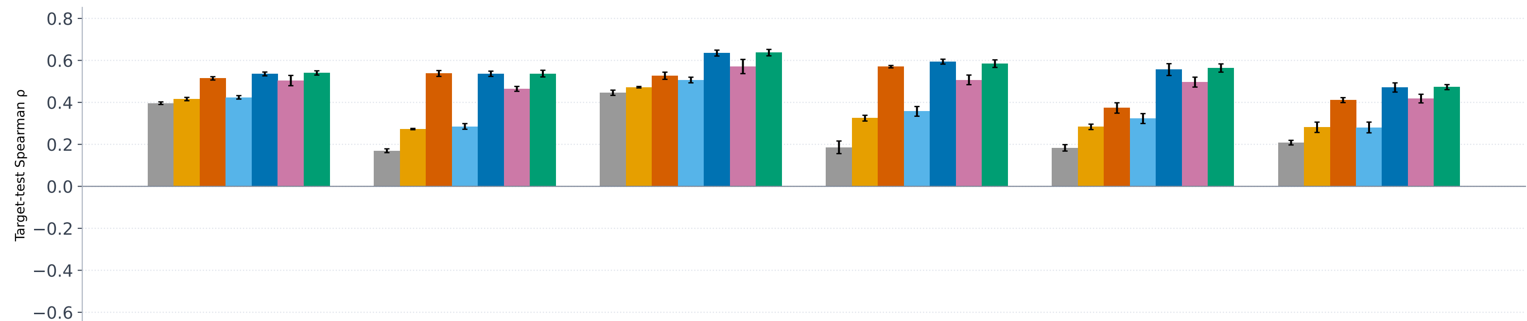
MLP
