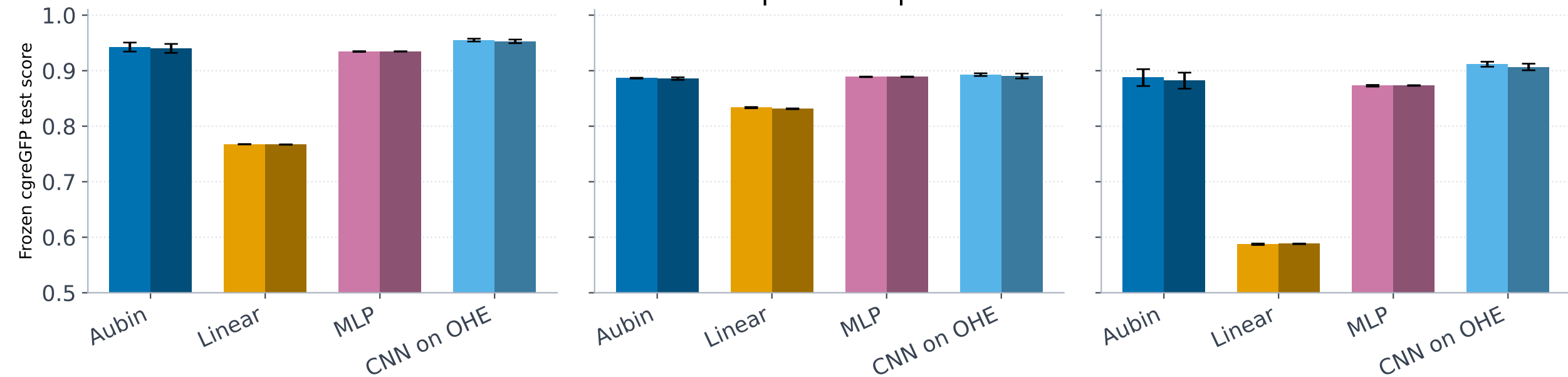
R^2
