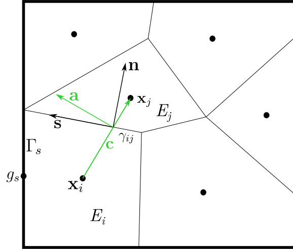
Рис. 2: Конечнообъёмная сетка
