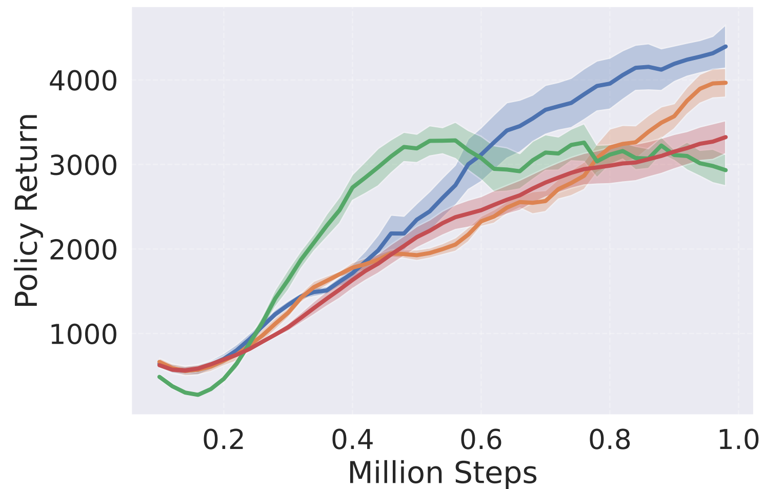
Ant-v5
