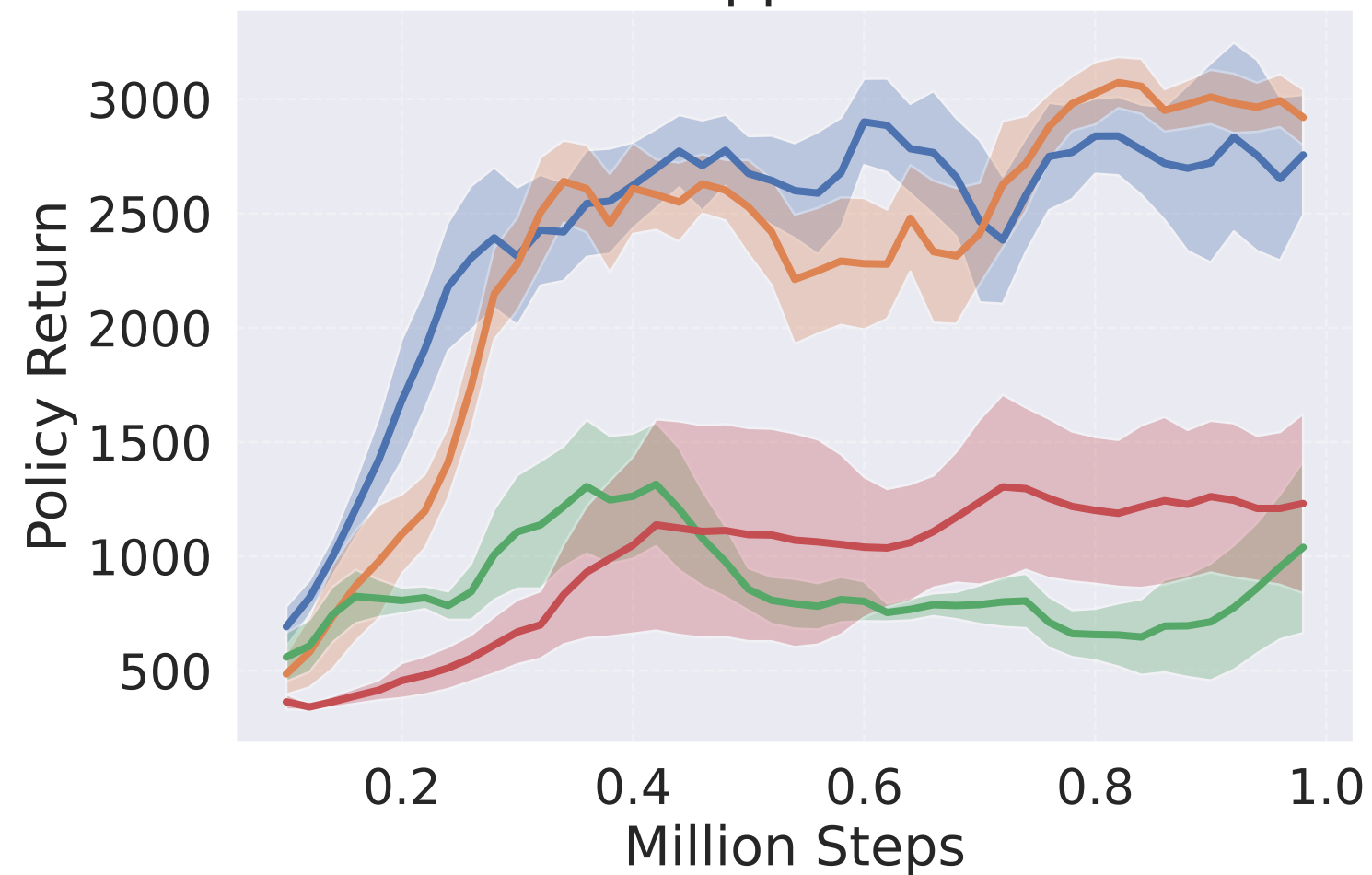
Hopper-v5
