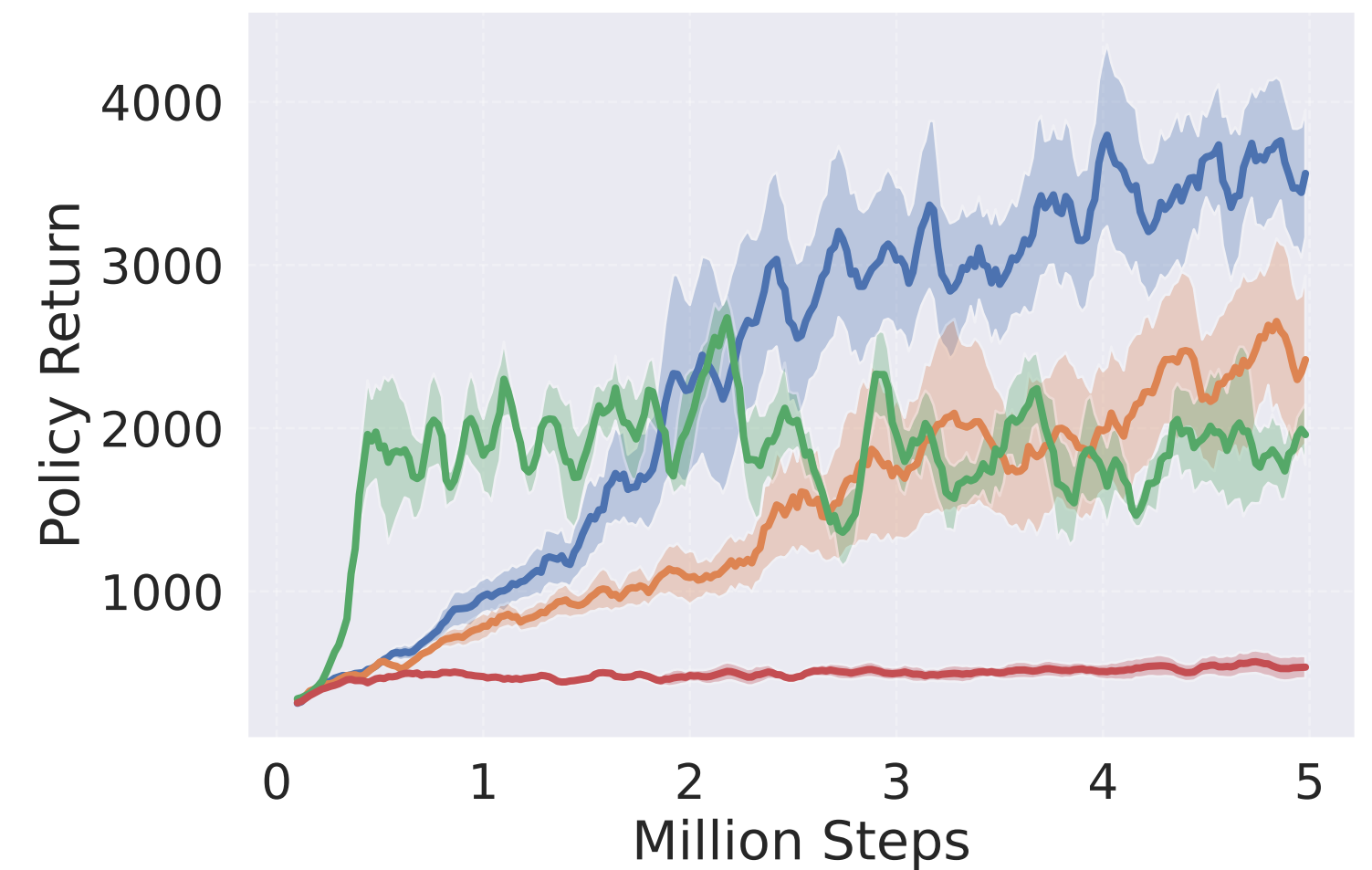
Humanoid-v5
