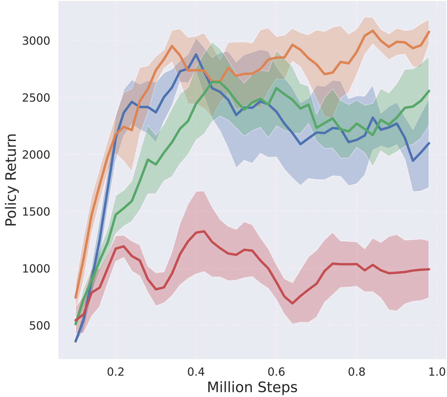
Hopper-v5
