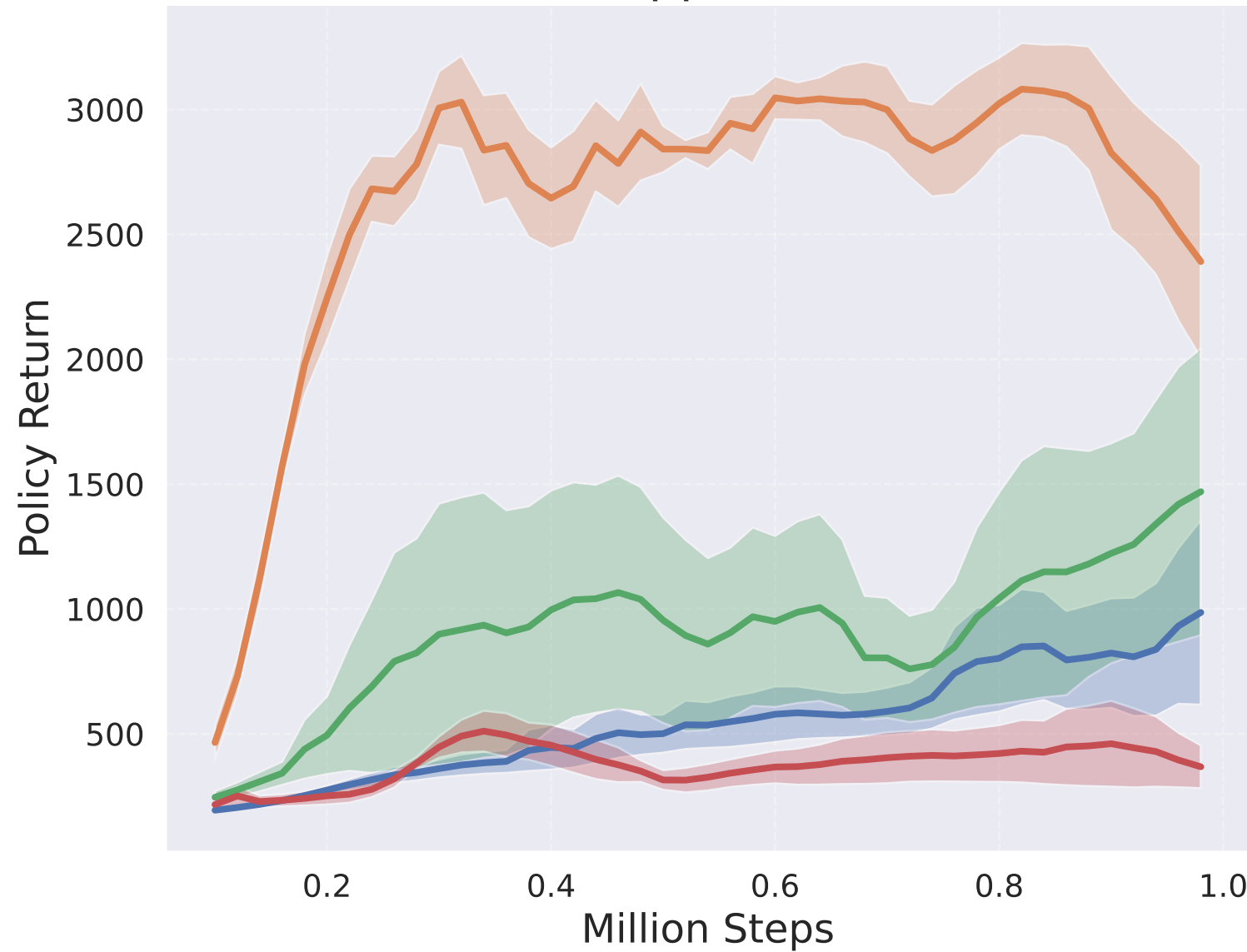
Hopper-v5
