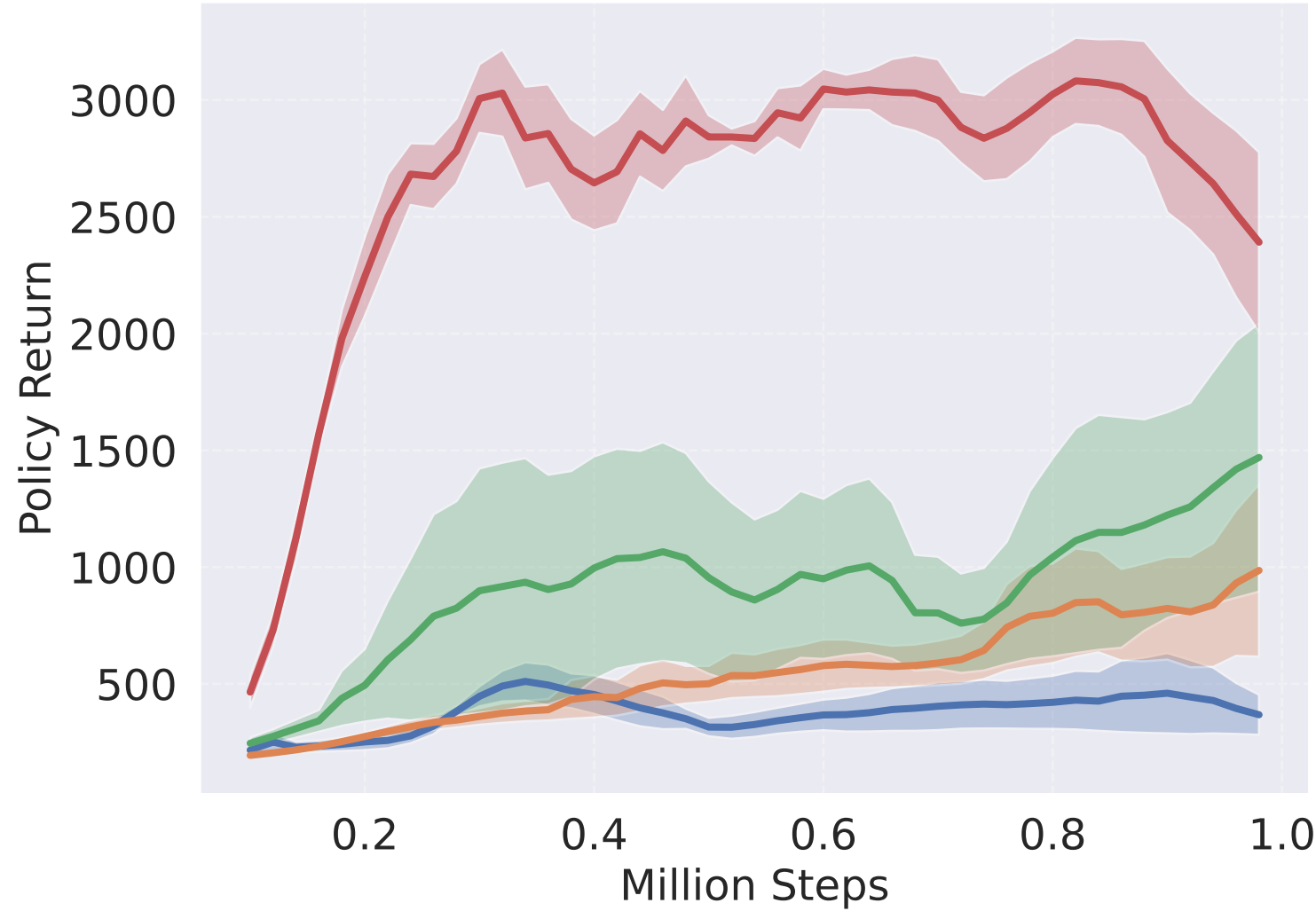
Hopper-v5
