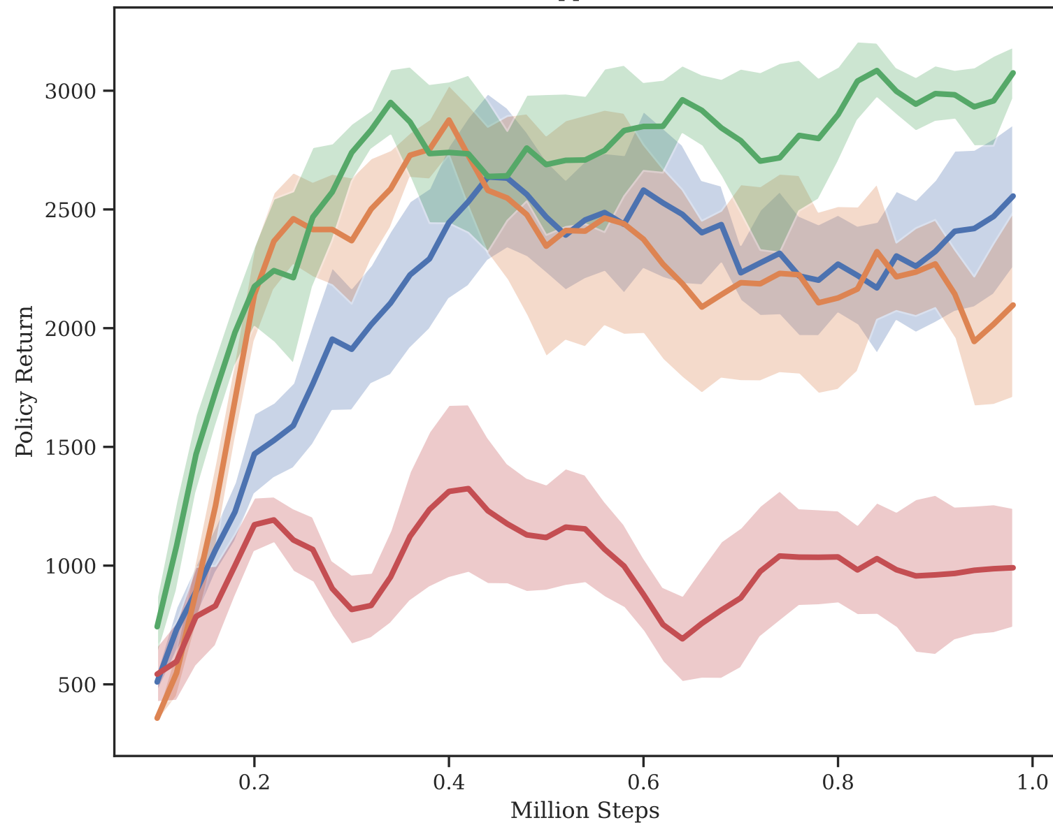
Hopper-v5
