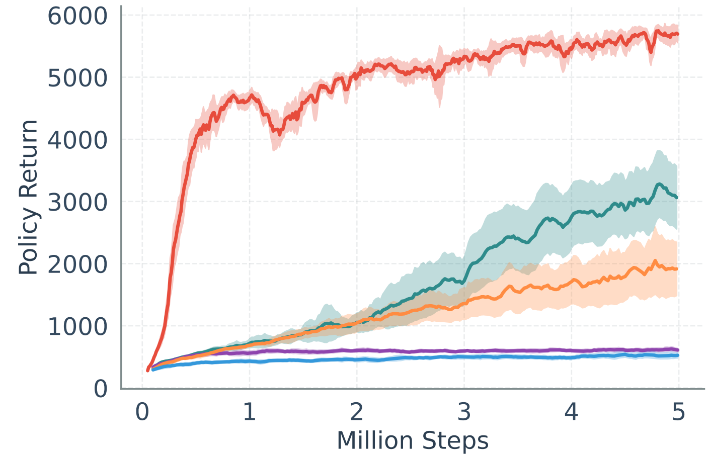
Humanoid-v5
