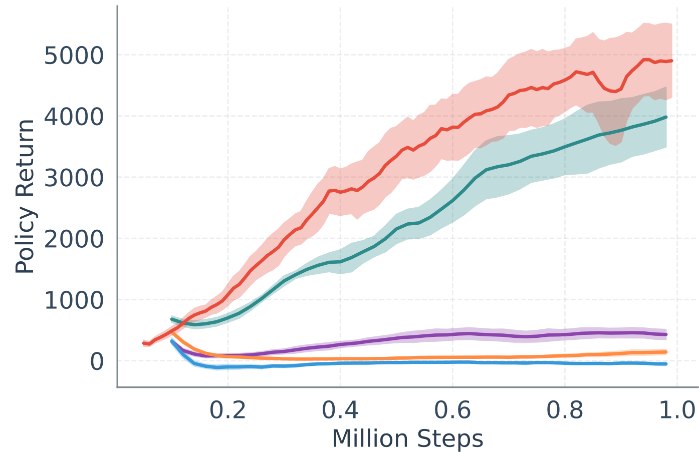
Ant-v5
