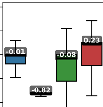
Ant
