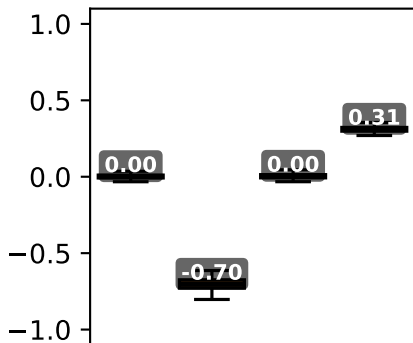
InvertedDoublePendulum
