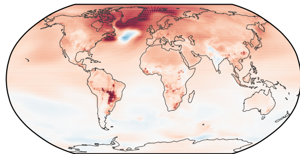
(a) CESM2
