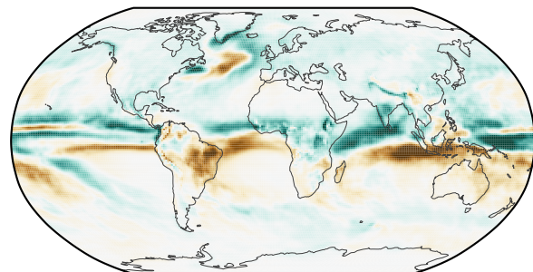
(a) CESM2
