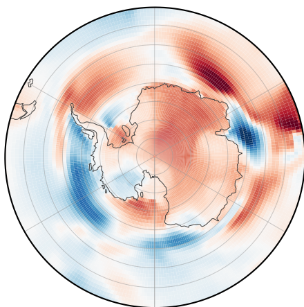
(d) CESM2 Antarctic mean +0.052\text{ }^{\circ}\text{C}
