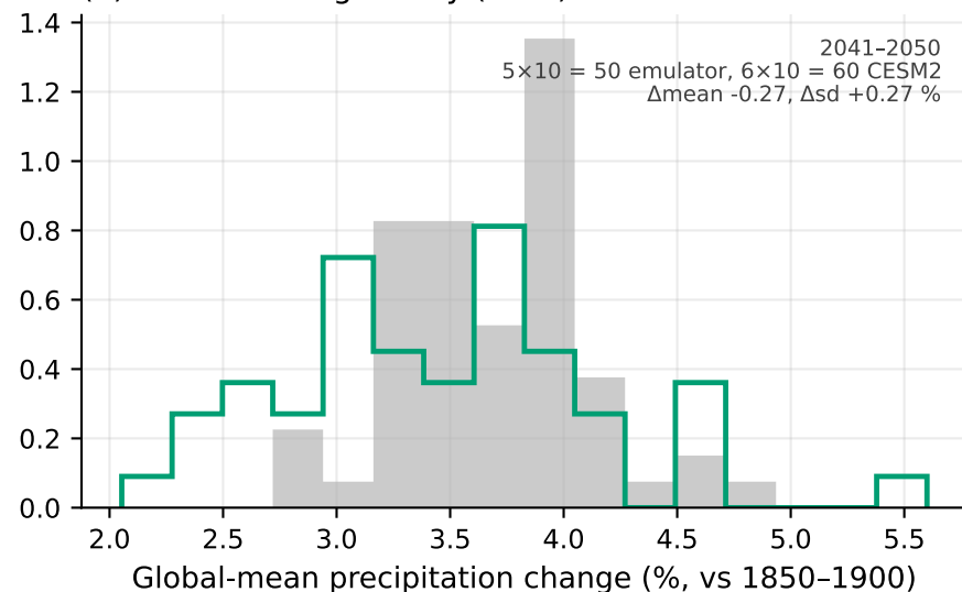
(d) Greenhouse-gas-only (GHG)
