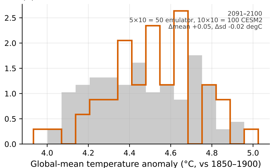
(d) Greenhouse-gas-only (GHG)
