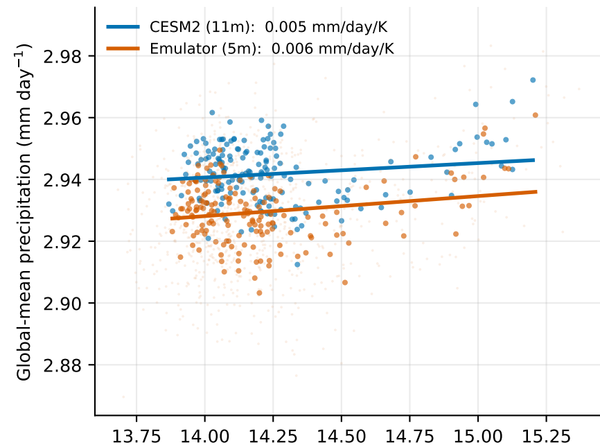
(d) GHG-only
