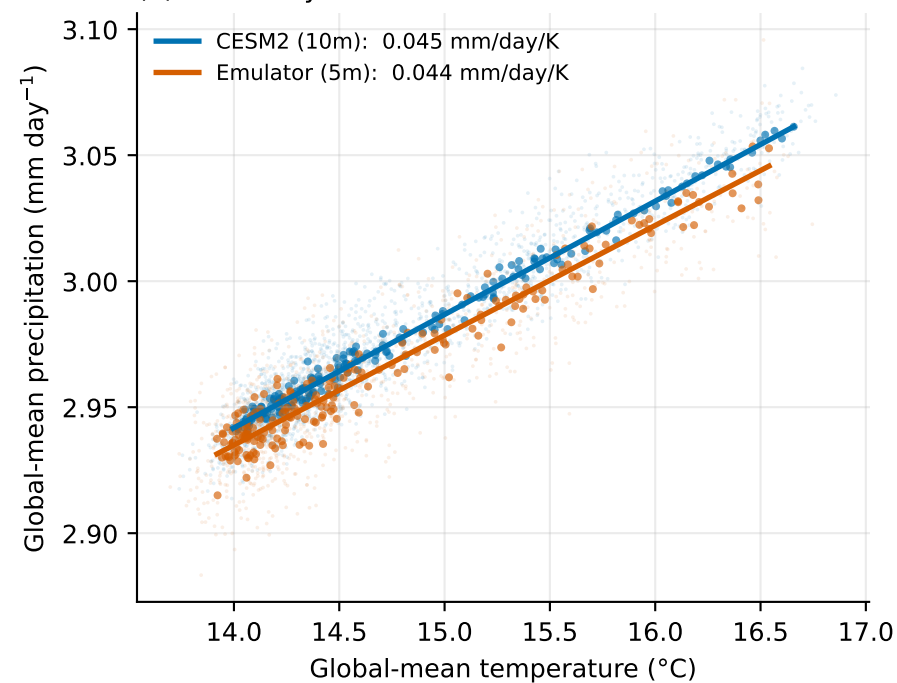
(d) GHG-only
