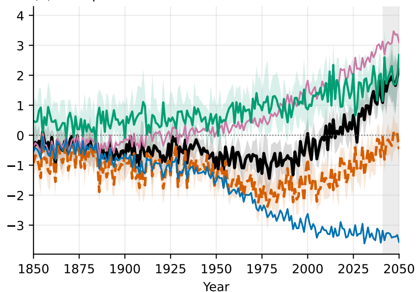
(d) Precipitation — Emulator
