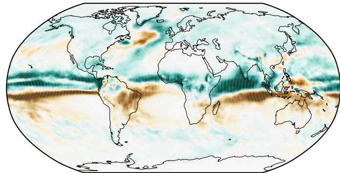
CESM2 R
