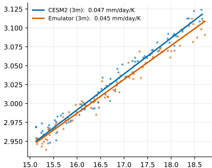
(d) GHG-only
