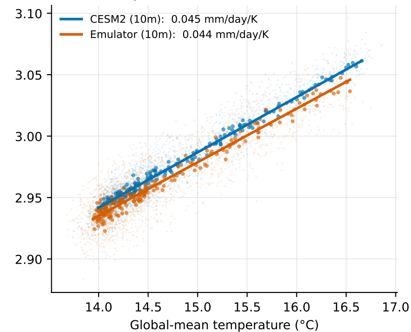
(d) GHG-only
