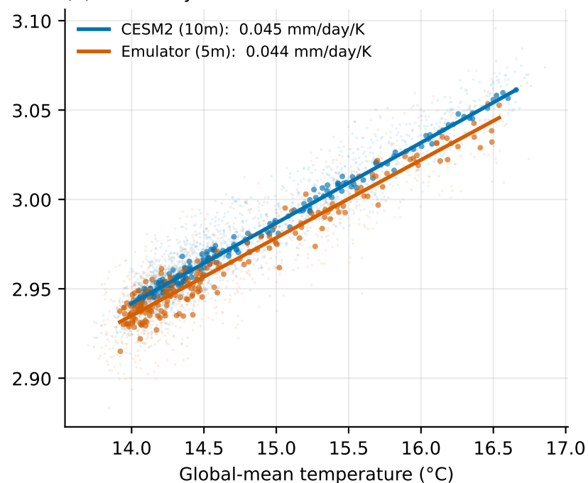
(d) GHG-only
