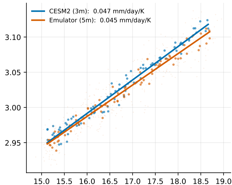
(d) GHG-only
