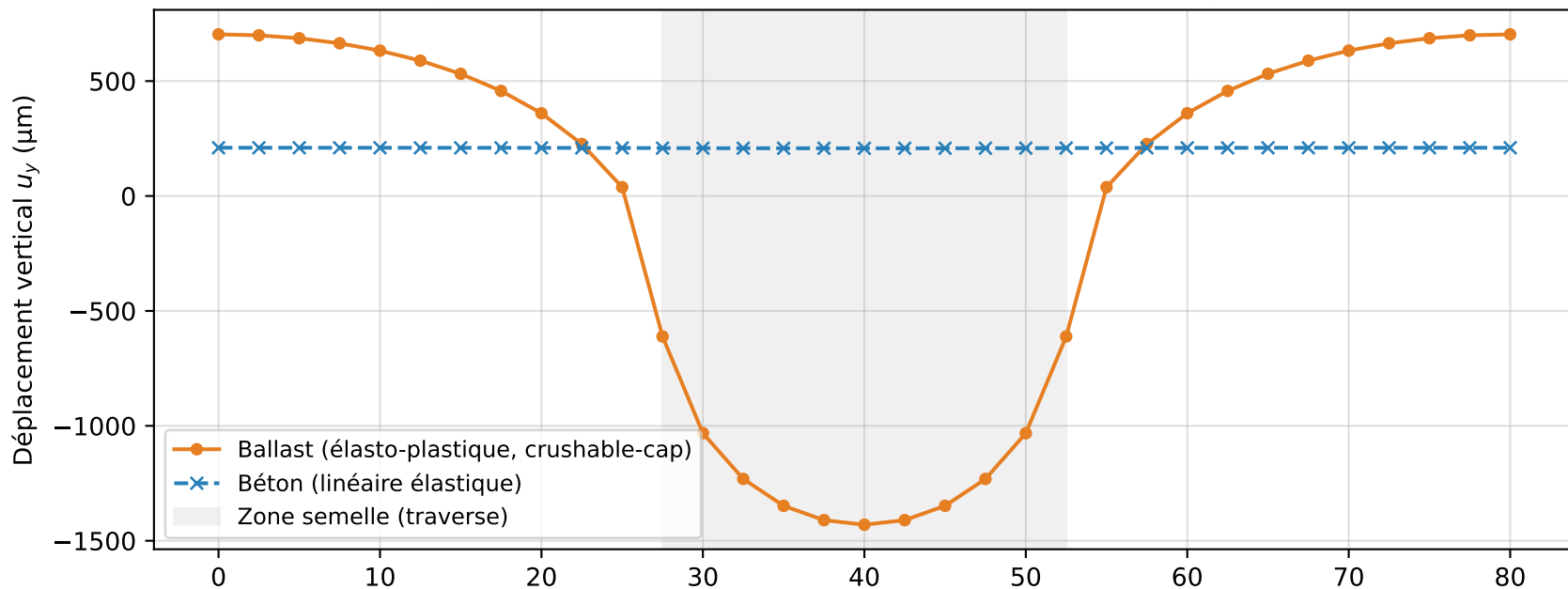
Réponse mécanique seule (soulèvement thermique retiré)
