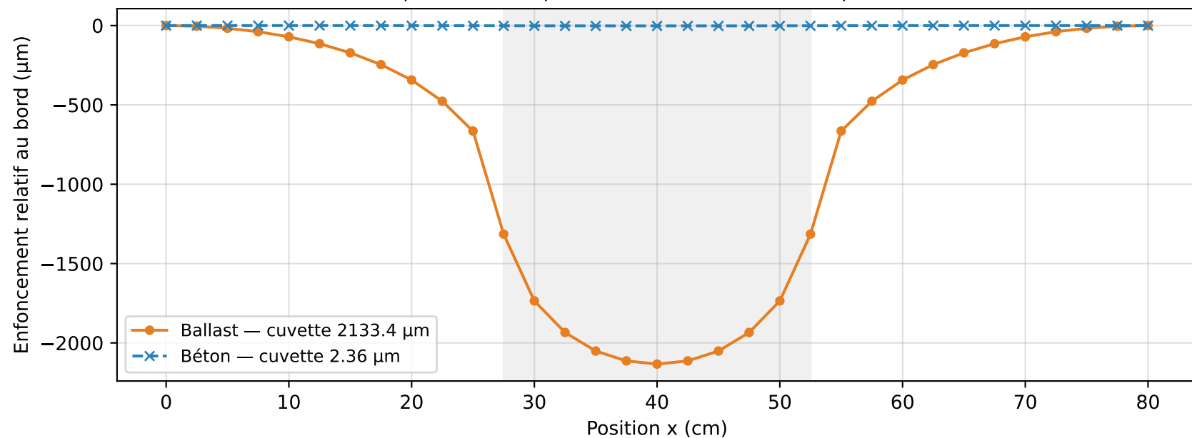
Réponse mécanique seule (soulèvement thermique retiré)
