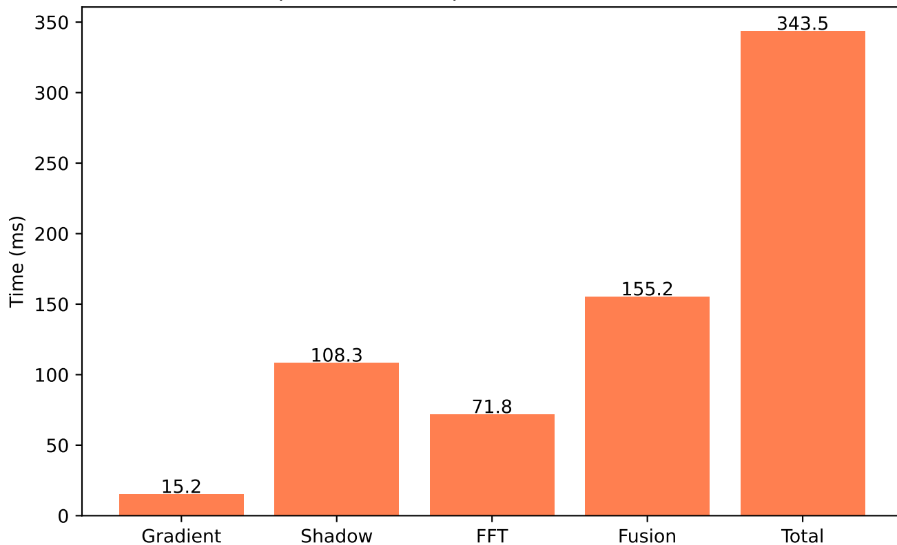
Pipeline Runtime per Module (1024x1024)
