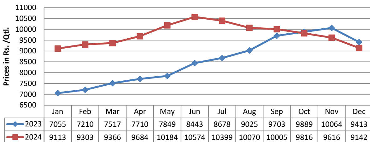
Fig. 37 अरहर (साबुत) Arhar (Whole)
