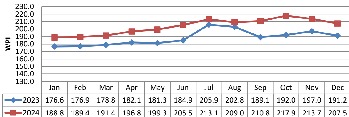
Fig. 57 खाद्य वस्तुओं के लिए WPI का संचलन Movement of WPI of Food Articles
