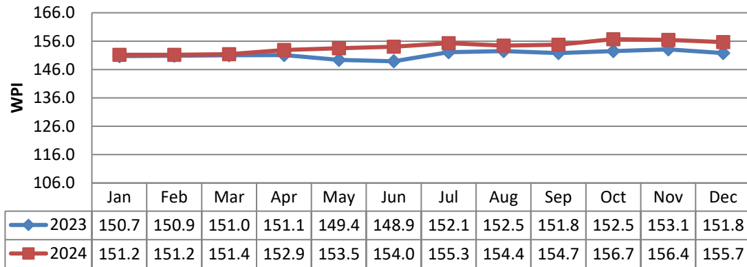
Fig. 55 सभी वस्तुओं के लिए WPI का संचलन Movement of WPI of All Commodities
