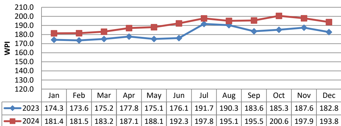
Fig. 56 प्राथमिक वस्तुओं के लिए WPI का संचलन Movement of WPI of Primary Articles
