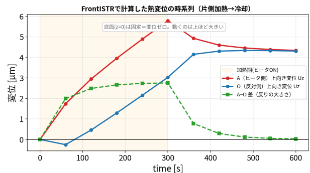
図 11: FrontISTR 真値の変位時系列
