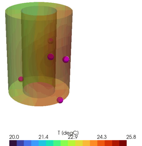
図 7: 5 点→全温度場の復元アニメ
