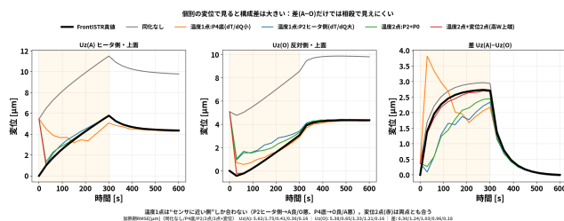
図 13: 個別の U_z(A)/U_z(O) と差の比較
