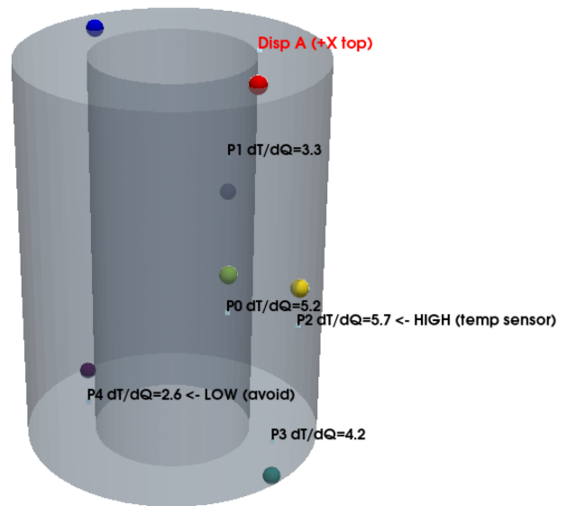
図 4: 5 温度点と変位観測点 A/O の位置
