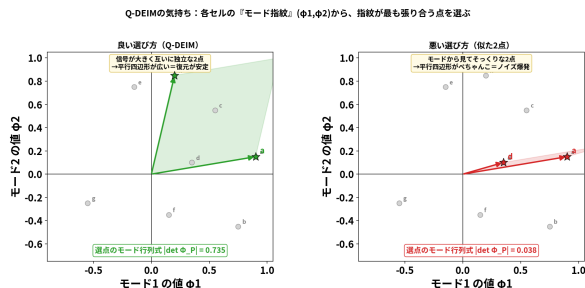
図 2: Q-DEIM の直感 (モード指紋と選点)
