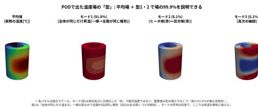
図 5: POD で出た温度場のモード
