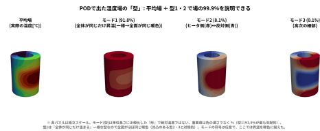
PODで出た温度場のモード
