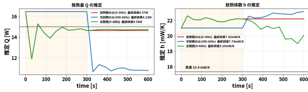
図 6: 同化時間窓の比較
