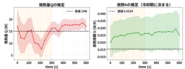
図 1: EnKF による Q \cdot h の推定
