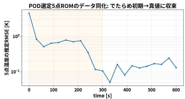
図 2: 温度 RMSE の収束
