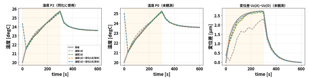
図 5: 段階比較の時系列
