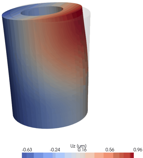
図 11: 熱変形のアニメーション
