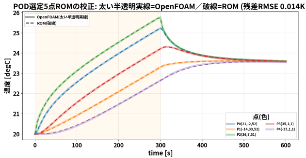
図 10: POD 選定 5 点 ROM の校正結果
