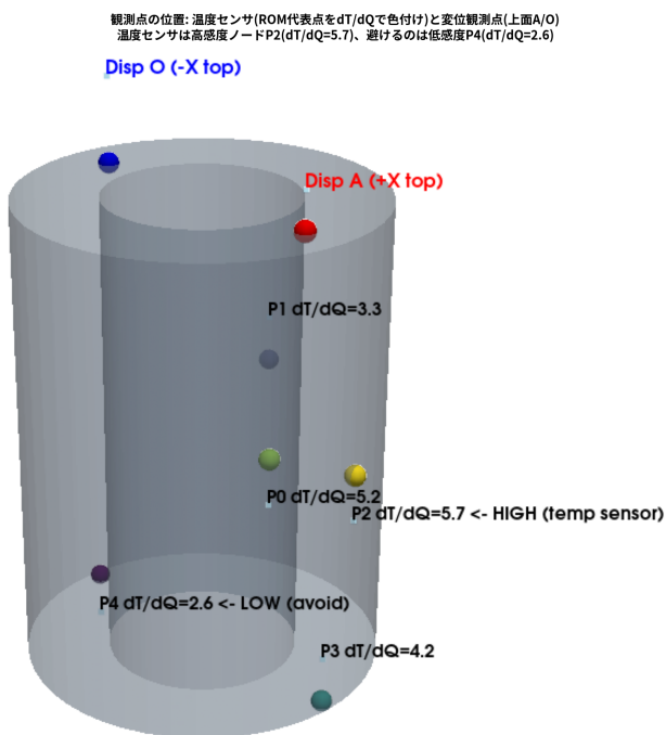
図 5: 5 温度点と変位観測点 A/O の位置
