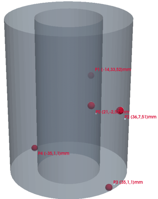
図 4: POD + Q-DEIM で選んだ ROM 代表点 (3D)
