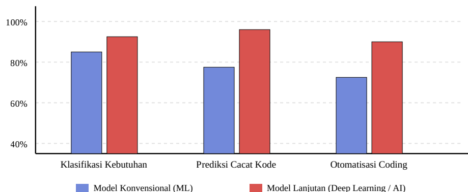
Gambar 2. Grafik Komparasi Tingkat Akurasi Eksperimental Algoritma Berdasarkan Dokumen SLR
