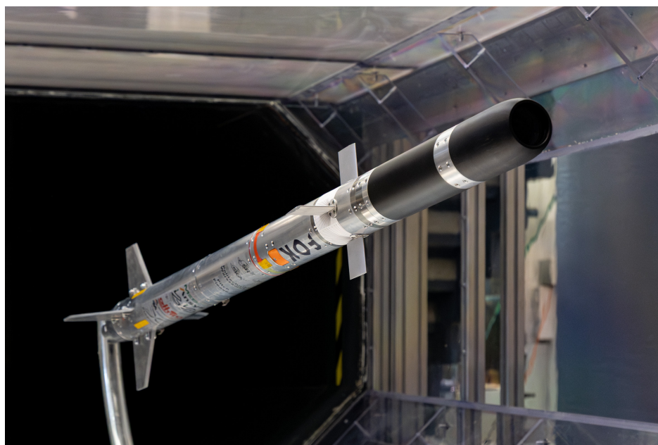
Rysunek 2.1. Rakieta FOK 2 w tunelu aerodynamicznym
