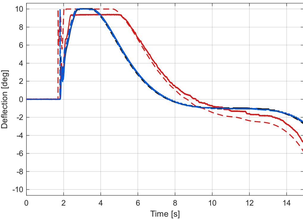
Canard 3
