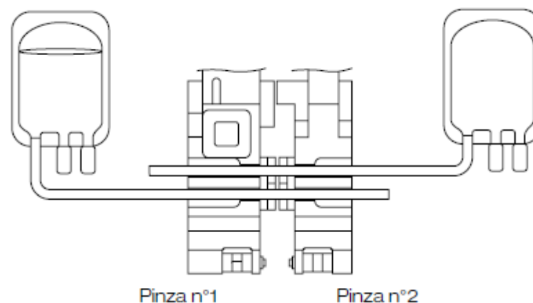
FIG 1 CORRECTA COLOCACION DE LAS TUBULADURAS
