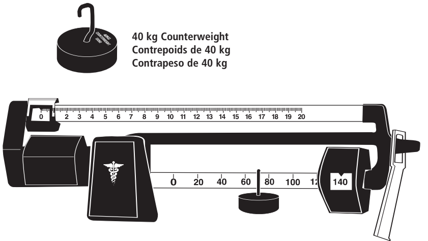
Placement of counterweight for patient over 180 kg Placement du contrepoids pour un patient pesant plus de 180 kg Colocación del contrapeso para un paciente que pesa más de 180 kg
