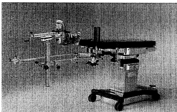
ALPHACLASSIC PRO con dispositivo de extensión para cirugía traumatológica.
