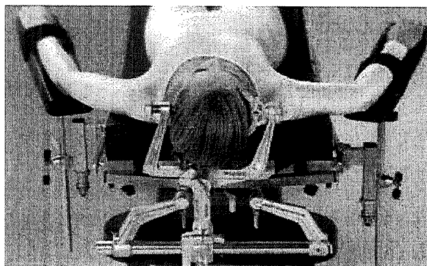
Posiciones muy bajas gracias al ajuste flexible de la parte superior de la mesa.
