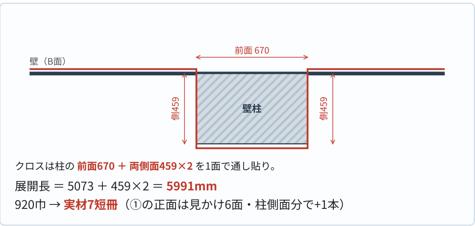
★ B面 壁柱の巻込（平面・拡大）
