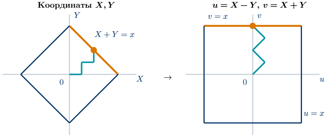
Рис. 4. При x = 4 путь RURU приводит к выходу (2, 2) , в новых координатах — (0, 4) . Оранжевая сторона X + Y = x становится границей v = x .
