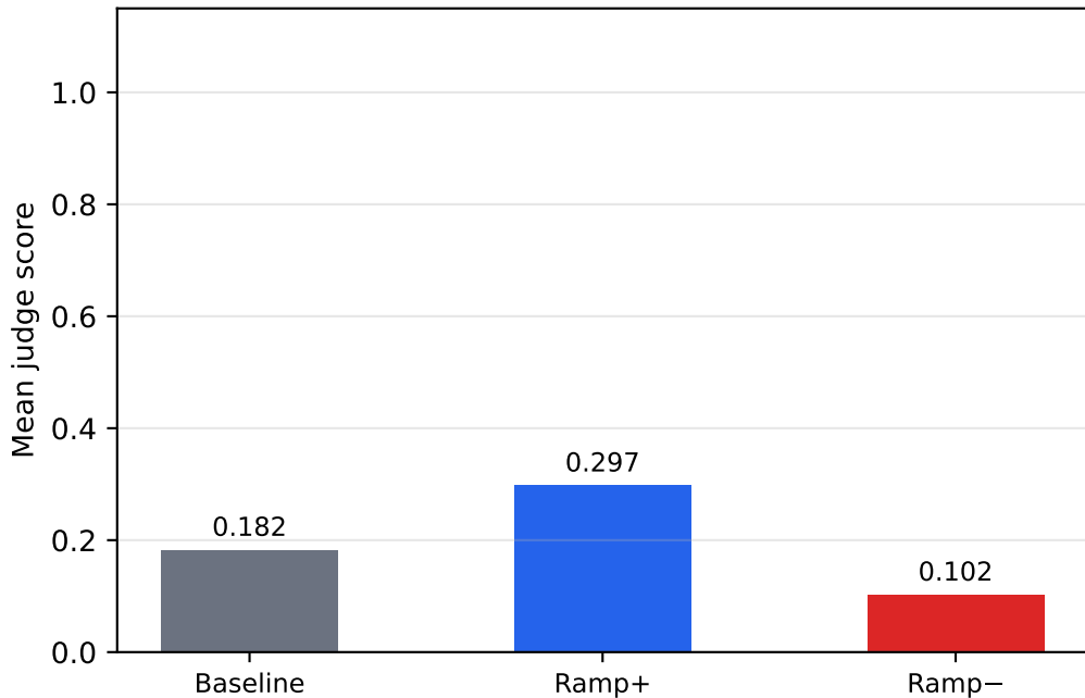
gemma-2-9b-it | sycophancy | k=1.00
