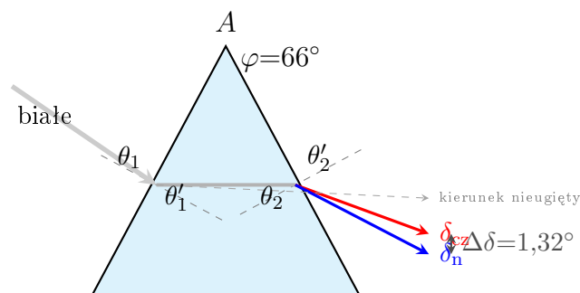
Rysunek 5: Rozszczepienie białego światła w pryzmacie szklanym ( n_{cz}=1,52 , n_n=1,54 , \varphi=66 ). Niebieskie (krótsze fale) odchyła się bardziej niż czerwone.
