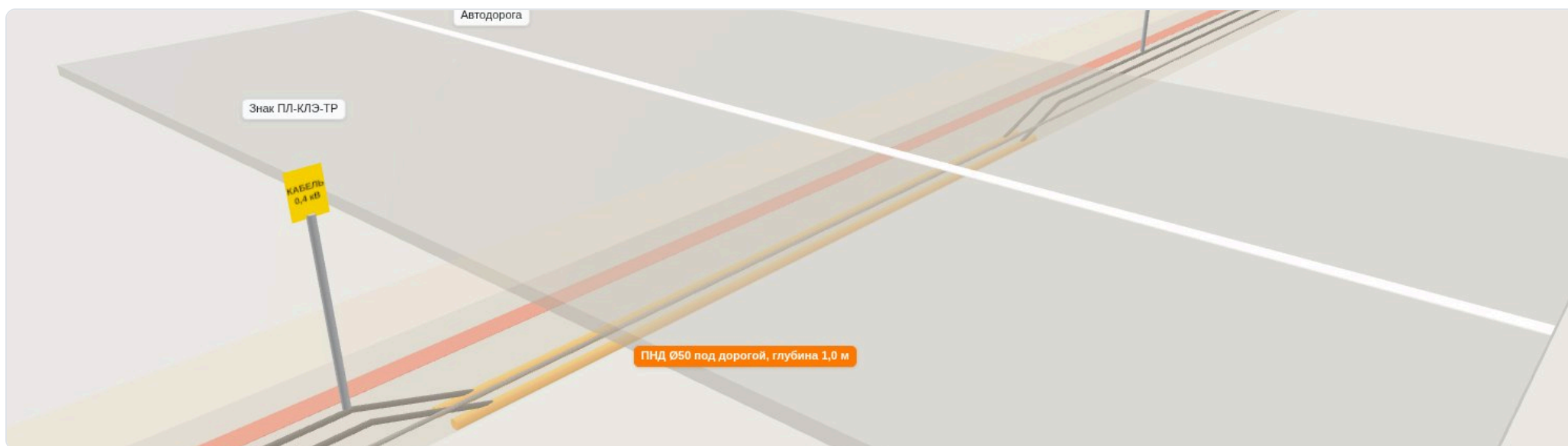
Рис. 6. Переход под автодорогой: две трубы ПНД Ø50 на глубине 1,0 м, концы уплотняются (эскиз 1, лист 7).
