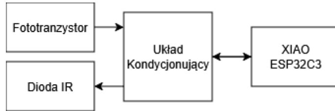
Rysunek 1. Diagram blokowy urządzenia
