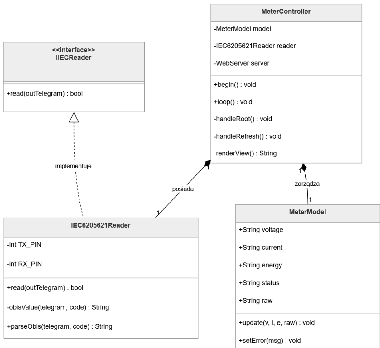
Rysunek 2. Diagram UML klas występujących w kodzie
